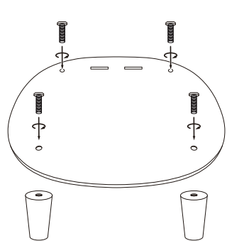
①脚を底板に取り付けます。
